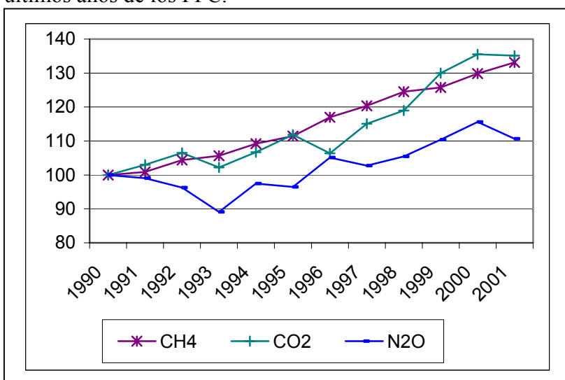
Figura 5. Evolución de las emisiones de gases de efecto invernadero (CO 2 , N 2 O y CH 4 ), 1990-2001. (1990=100)
