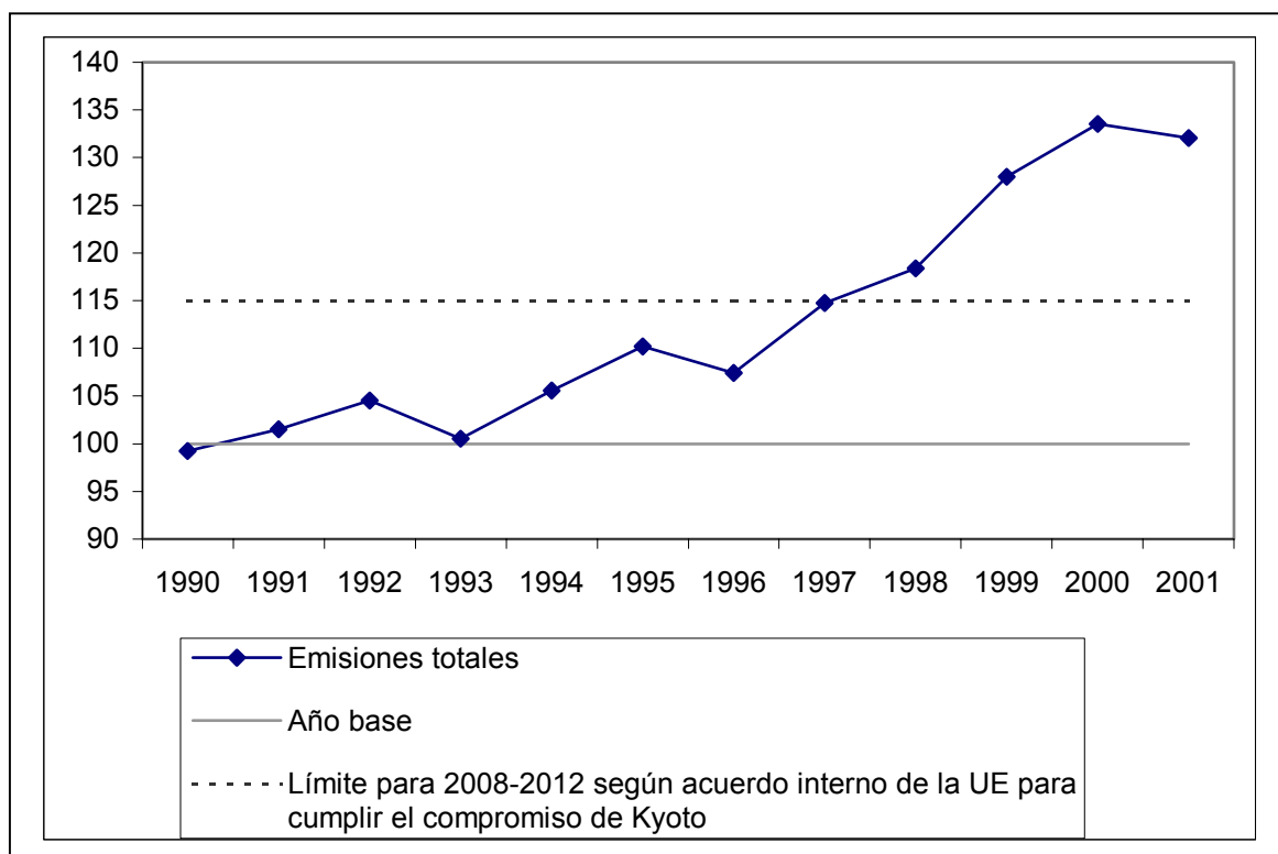
Figura 7. Evolución de las emisiones totales de CO 2 -equivalente, 1990-2001 respecto al año base del protocolo de Kyoto.
