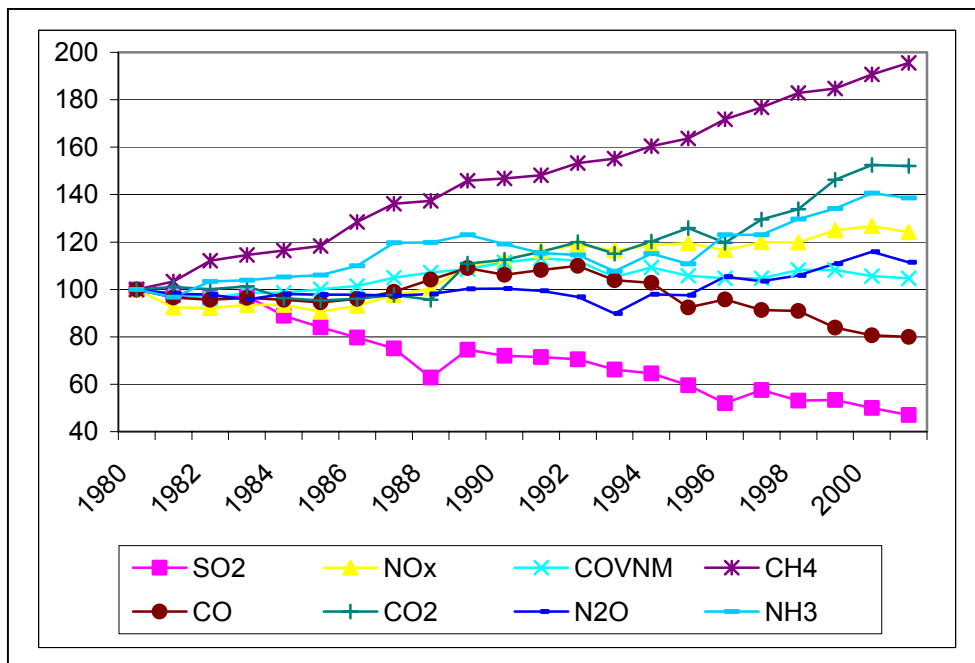
Figura 2. Evolución de las emisiones en España, 1980-2001 (1980=100)
