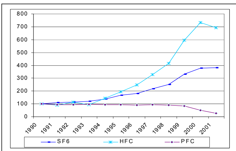
Figura 6. Evolución de las emisiones de gases de efecto invernadero (SF 6 , HFC y PFC), 1990-2001
